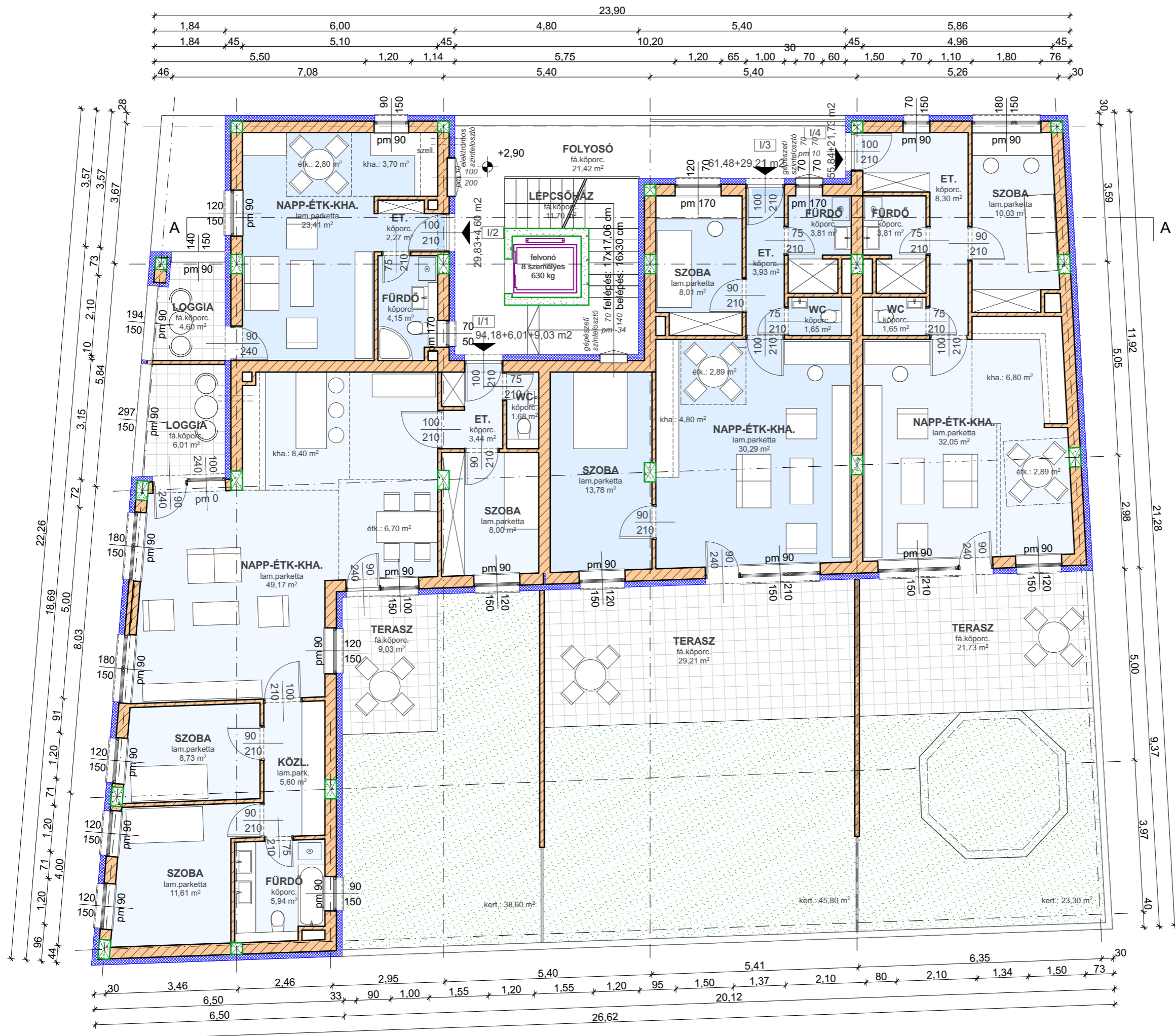
I. EMELETI ALAPRAJZ - M = 1:100
