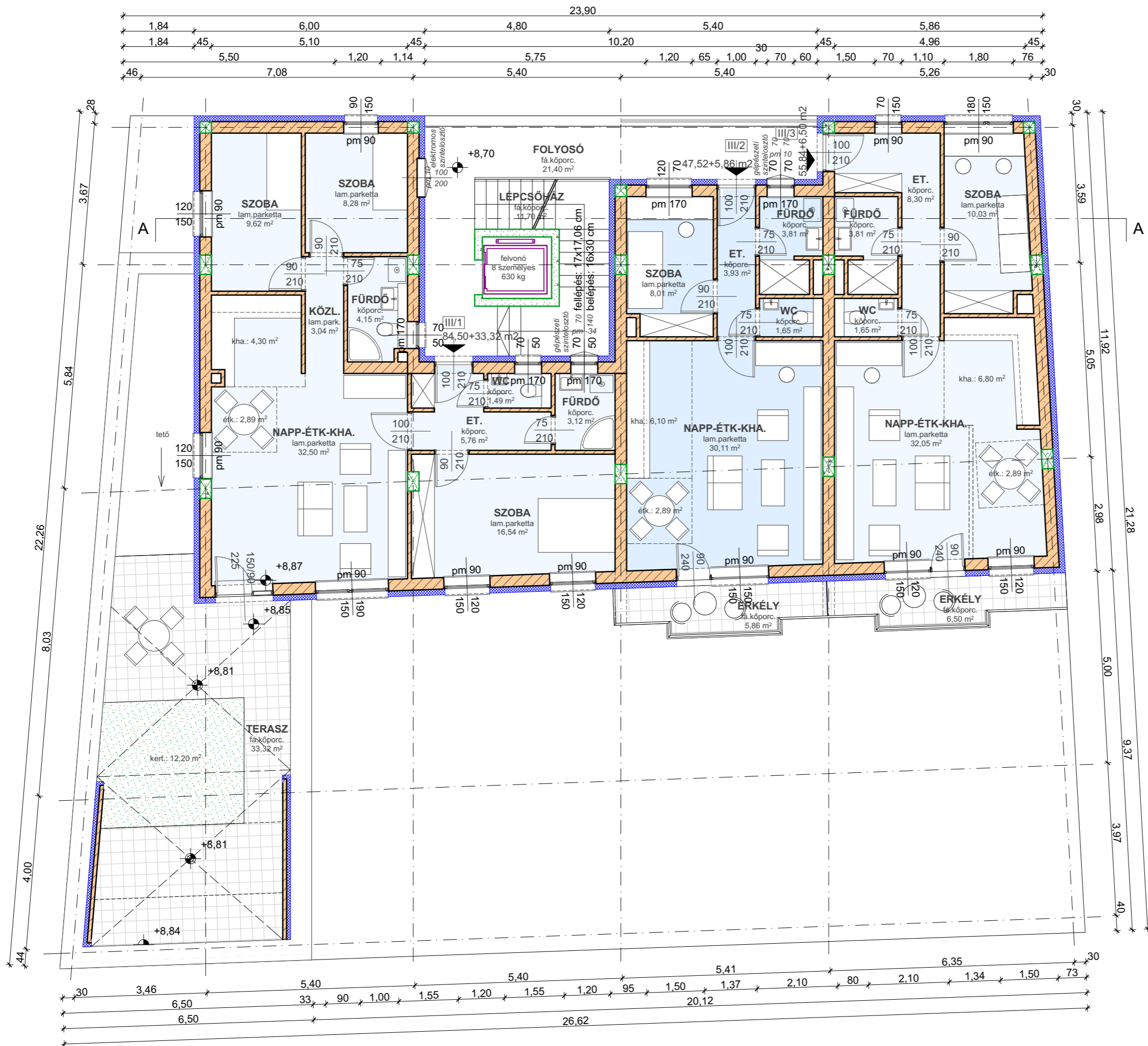
III. EMELETI ALAPRAJZ - M = 1:100
