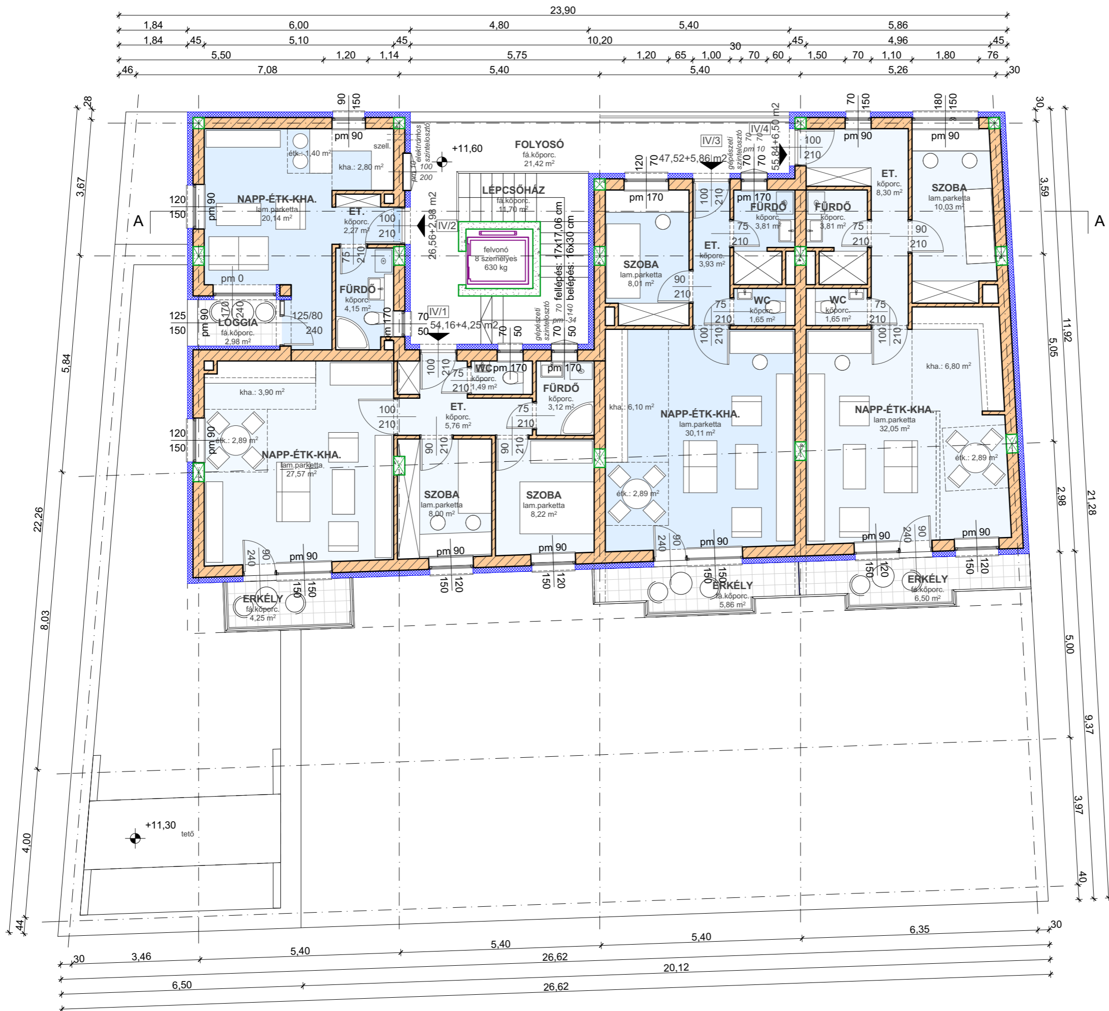
IV. EMELETI ALAPRAJZ - M = 1:100
